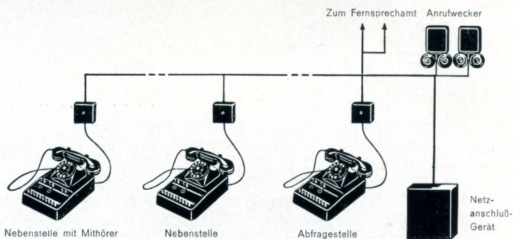
Schema einer Reihenanlage für 2 Amtsleitungen und 10 Nebenstellen
