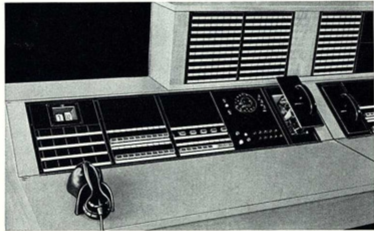
Belegzetteldrucker für die Aufzeichnung der Gesprächsgebühren und -daten in den Vermittlungsplätzen einer TuN-Universalzentrale
