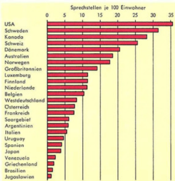
Die Sprechstellendichte verschiedener Länder (Stichtag 1. 1. 1957)
