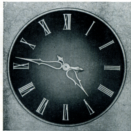
Nr. 431 23/8 Patina-Zifferblatt, nach außen dunkel verlaufend; Zeiger, Zahlen und Zierreif aus Messing 30, 40, 50 und 60 cm \phi
