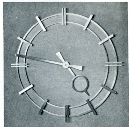
Nr. 431 23/6 * Elfenbeinfarbiges Zifferblatt; Zeiger, Ringe und Keile aus Messing 30, 40, 50, 60, 80 und 100 cm \phi
